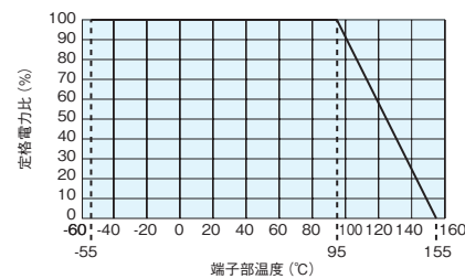
端子部温度 WU73 2B15 (1.5W)
