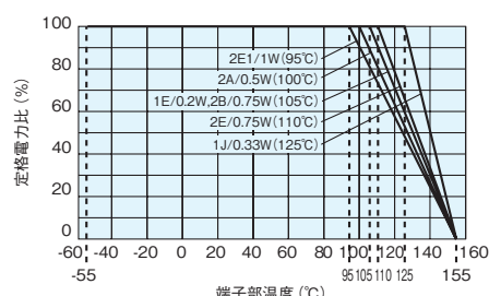
端子部温度
