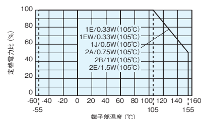
端子部温度
