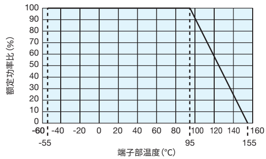
端子部温度
